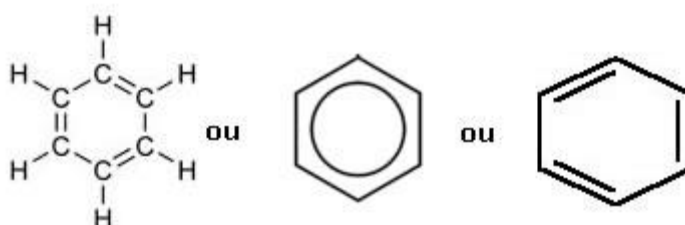
Figura 3.4 – Anel benzênico.
